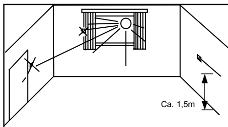
Fig. 2.a Rumtermostatens placering
