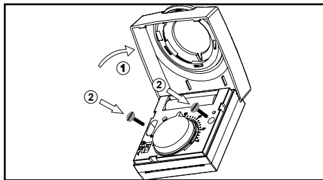
Fig. 2.b Rumtermostatens montering
